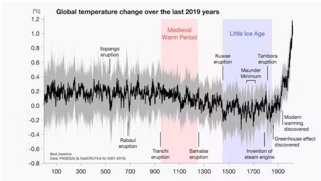
Températures moyennes globales depuis l'an 0. Ed Hawkins
